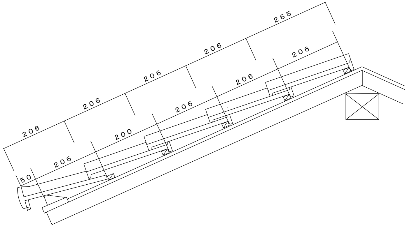
越前瓦 流れ7 2判割付け
